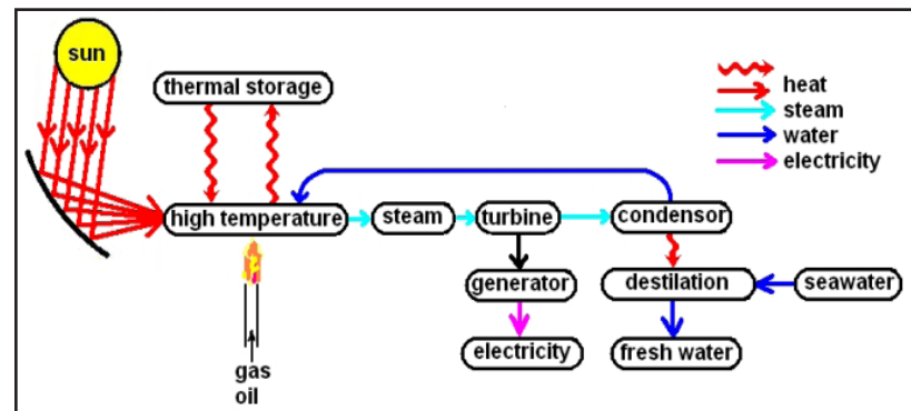
رسم توضيحي لألية توليد الكهرباء من أشعة الشمس المركزة
